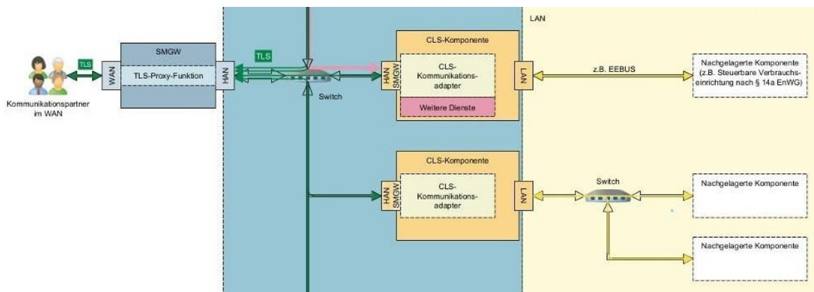
Abbildung 13: CLS-Komponenten an der SMGW-HAN-Schnittstelle (Quelle: TR 03109-5)
