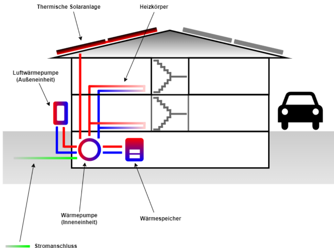
Abbildung 2: Übersicht Wärmeerzeugung und -verteilung
