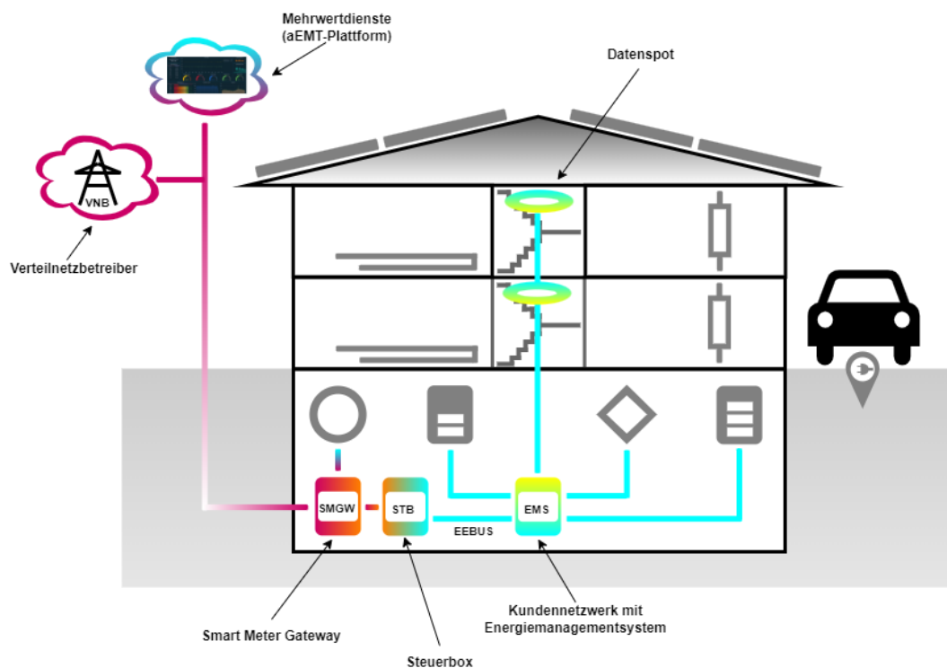
Abbildung 12: Übersicht Datenquellen/senken und -verteilung
